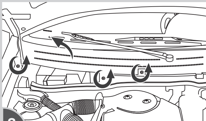
3 REMOVER 3 TORNILLOS Y RETIRAR CUBIERTA IZQUIERDA
