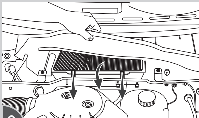
6 DESENGANCHAR Y CAMBIAR EL FILTRO
