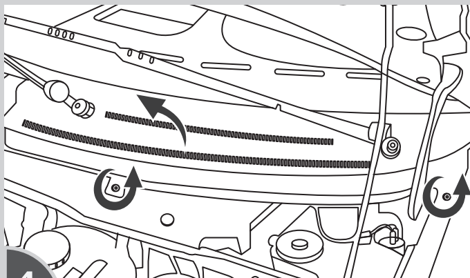
4 REMOVER 2 TORNILLOS Y RETIRAR CUBIERTA DERECHA
