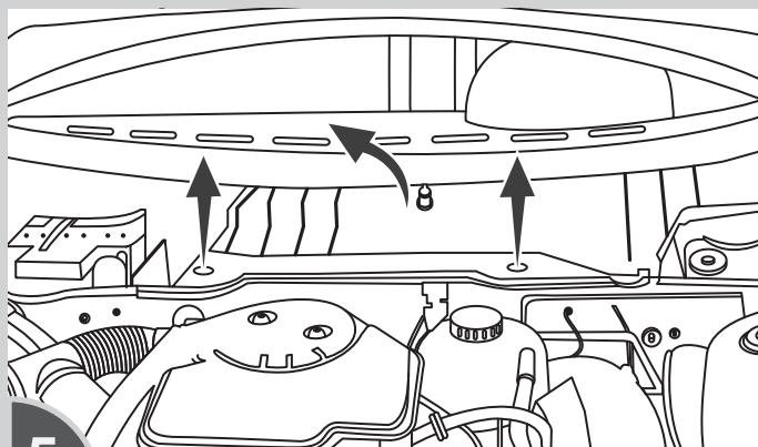
5 DESENGANCHAR Y RETIRAR LA CUBIERTA CENTRAL
